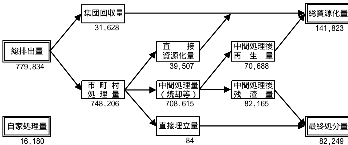
図 ごみ処理のフロー (平成16年度)
